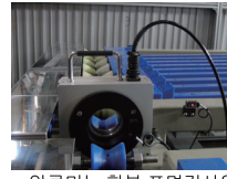
* 알루미늄 환봉 표면검사용 관통식 프로브
